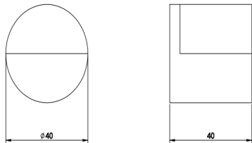
Door stop | DS0026
